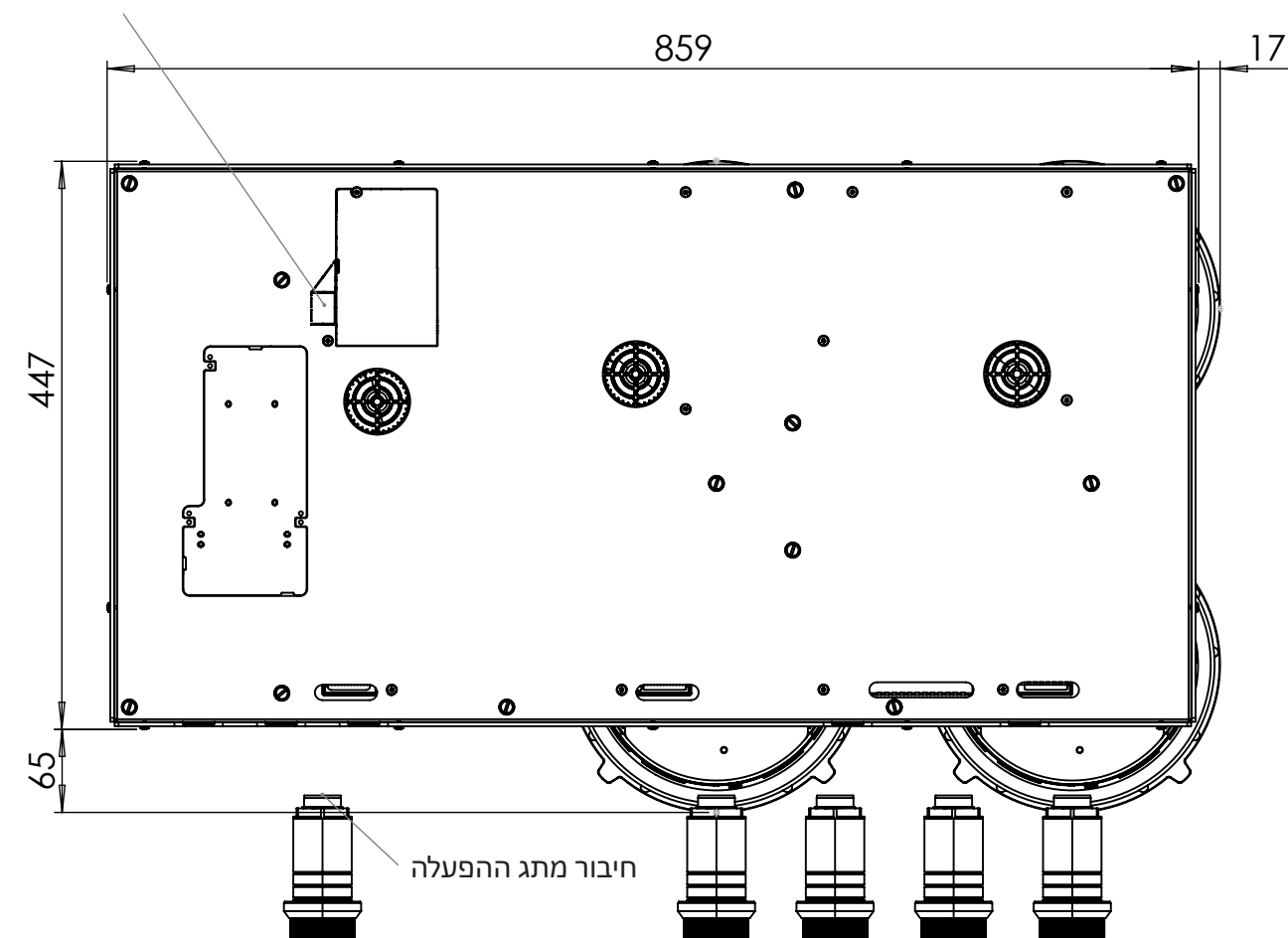
מבט תחתון
