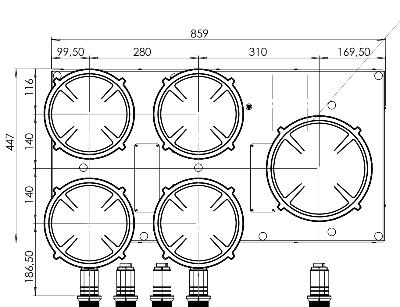
מבט עליון
