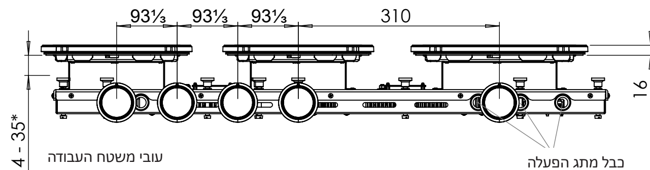
מבט חזיתי
